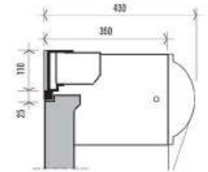
SEZIONE VERTICALE VERTICAL SECTION
