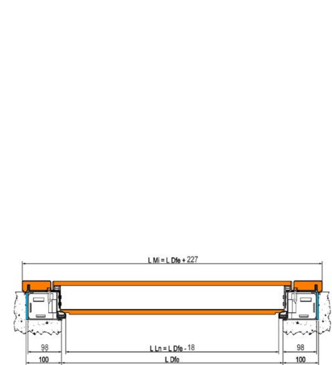
SOPRALZO FISSO CIECO IN PANNELLO (STESSA FINITURA DELL'ANTA) / FIXED TRANSOM (SAME FINISHING AS THE DOOR)
