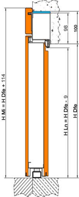
LATERALE FISSO CIECO IN PANNELLO (STESSA FINITURA DELL'ANTA) / FIXED LATERAL PANEL (SAME FINISHING AS THE DOOR)
