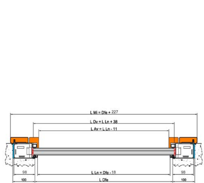
SOPRALZO FISSO PREDISPOSTO PER VETRO / FIXED TRANSOM PREPARED FOR GLASS
