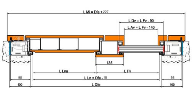
LATERALE FISSO PREDISPOSTO PER VETRO / FIXED LATERAL PREPARED FOR GLASS
