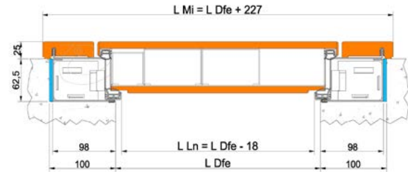
SEZIONE ORIZZONTALE HORIZONTAL SECTION
