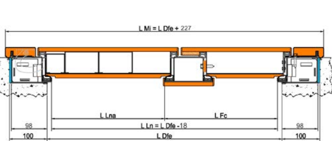
LATERALE FISSO CIECO IN PANNELLO (STESSA FINITURA DELL'ANTA) / FIXED LATERAL PANEL (SAME FINISHING AS THE DOOR)
