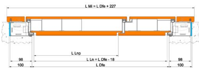
SEZIONE ORIZZONTALE - 2 ANTE HORIZONTAL SECTION - 2 LEAVES
